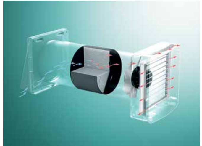
Rekuperacija topline kroz keramički izmjernjivač topline
